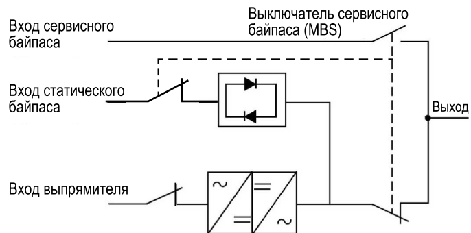
Рис. 7-9: Режим двойного преобразования
