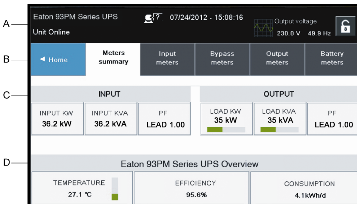
Рис. 7-1: Компоненты дисплея
