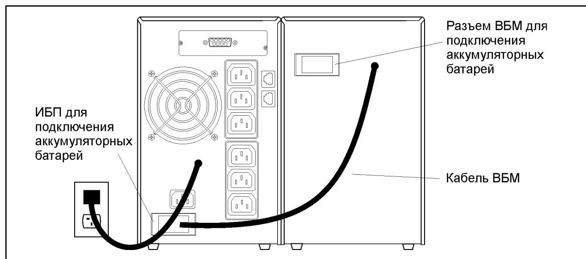
Рисунок 12. Подключение ВБМ
