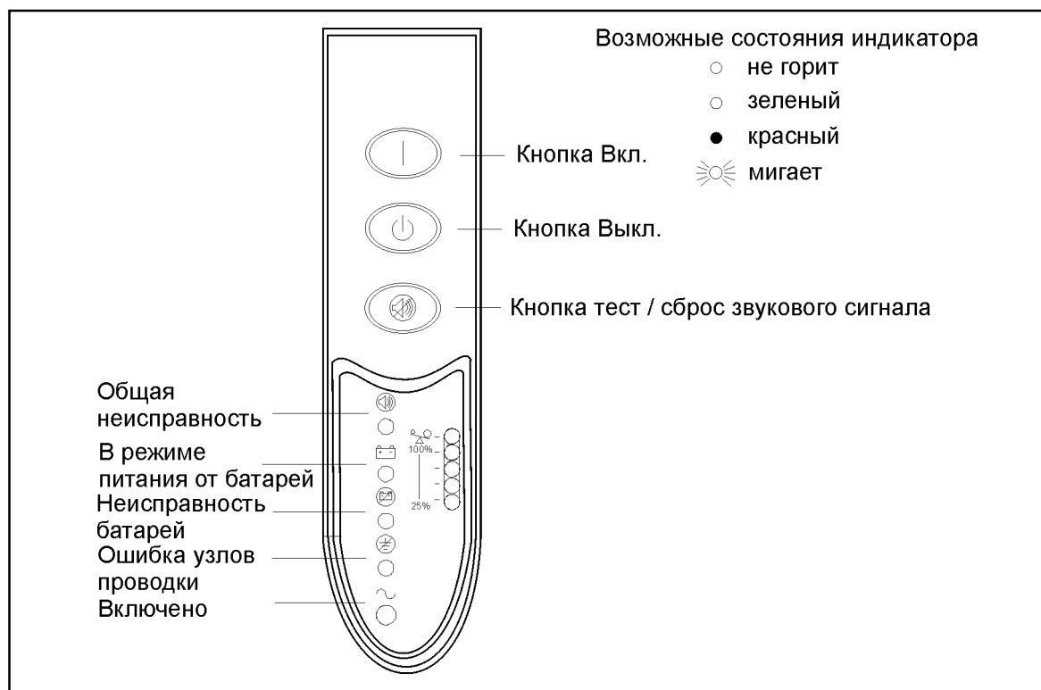
Рисунок 13. Индикаторы тревоги.
